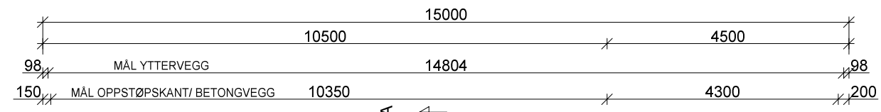
FASADE VEST
