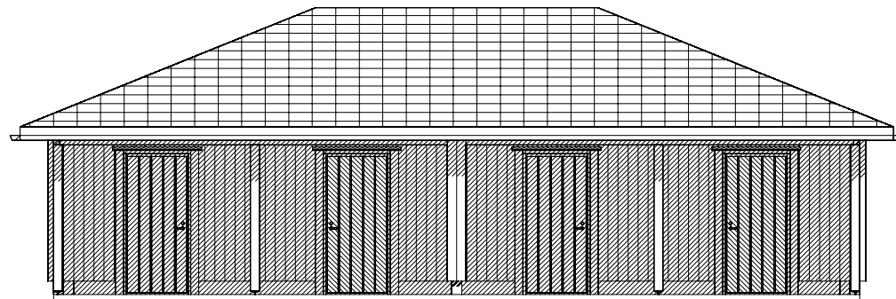
FASADE ØST
