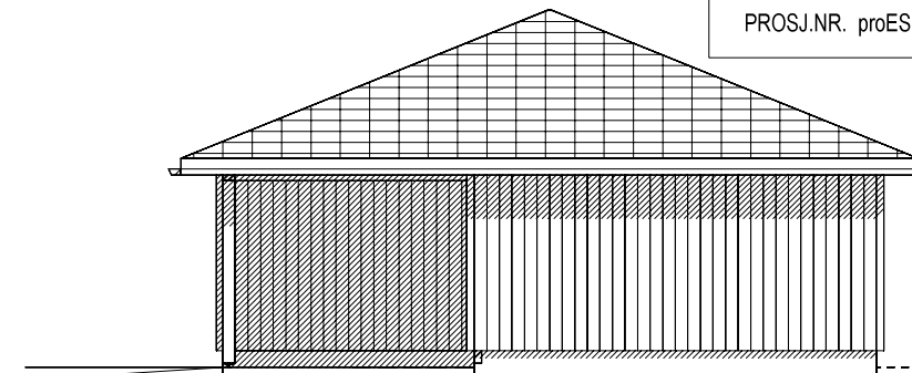
FASADE NORD
